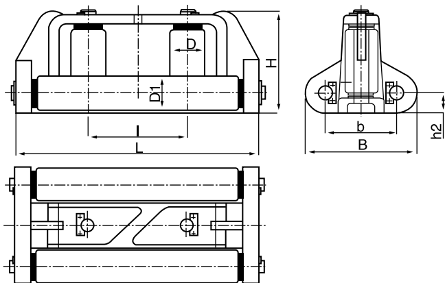
工程船导缆器 B型 Engineering ship' s fairlead Type B CB*3015-83
